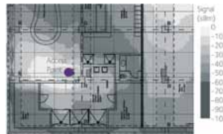
Ausleuchtung Wellenbereich/Hotel (0 dBm beste Signalstärke, -60 dBm noch akzeptabel)
